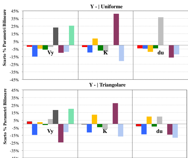
Figura 8. Scarto percentuale rispetto al valore medio delle tre grandezze che definiscono la bilineare equivalente.
