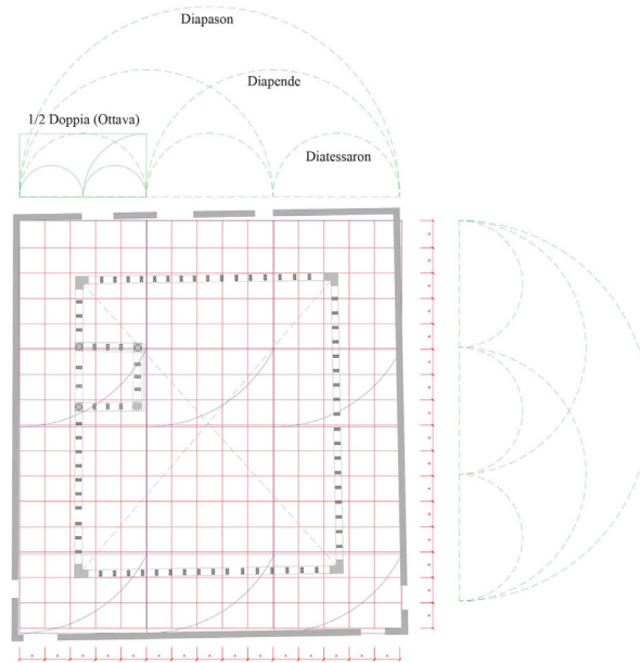
Modulo "A" costruito sul lato più corto del rettangolo di base
