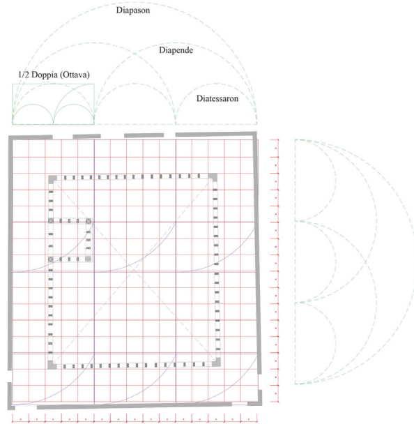
Modulo "A" costruito sul lato più corto del rettangolo di base
