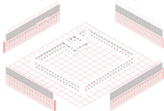
Moduli geometrici nel modello tridimensionale
