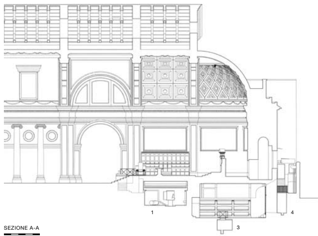
SEZIONE A-A 0 5m
